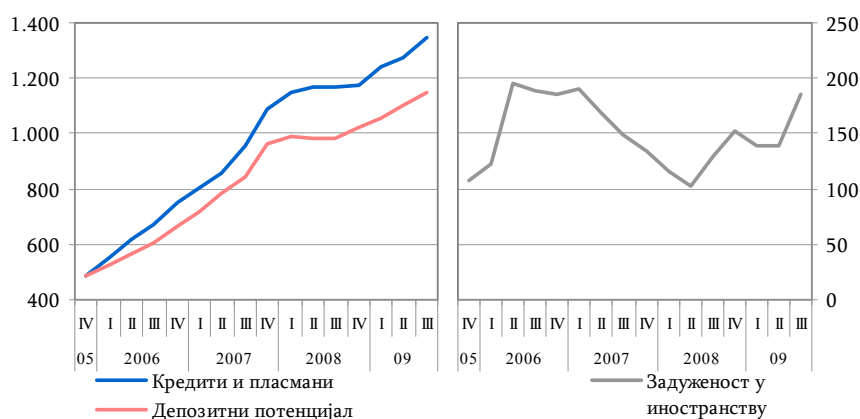
Графикон 4. Кредити 8 , депозити и кредитна задуженост банака
