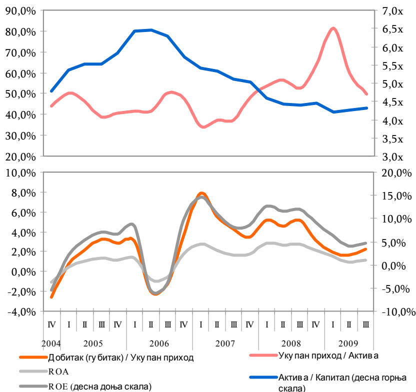
Графикон 10. DuPont декомпозиција профитабилности банкарског сектора (Децембар 2004 – Септембар 2009)
