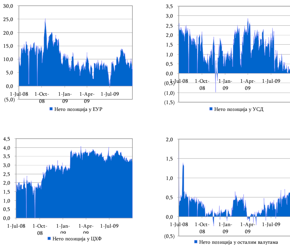
Графикон 7. Приказ кретања нето отворене позиције у одређеним валутама за период јул 2008 – септембар 2009.
